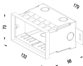
pot d'encastrement
